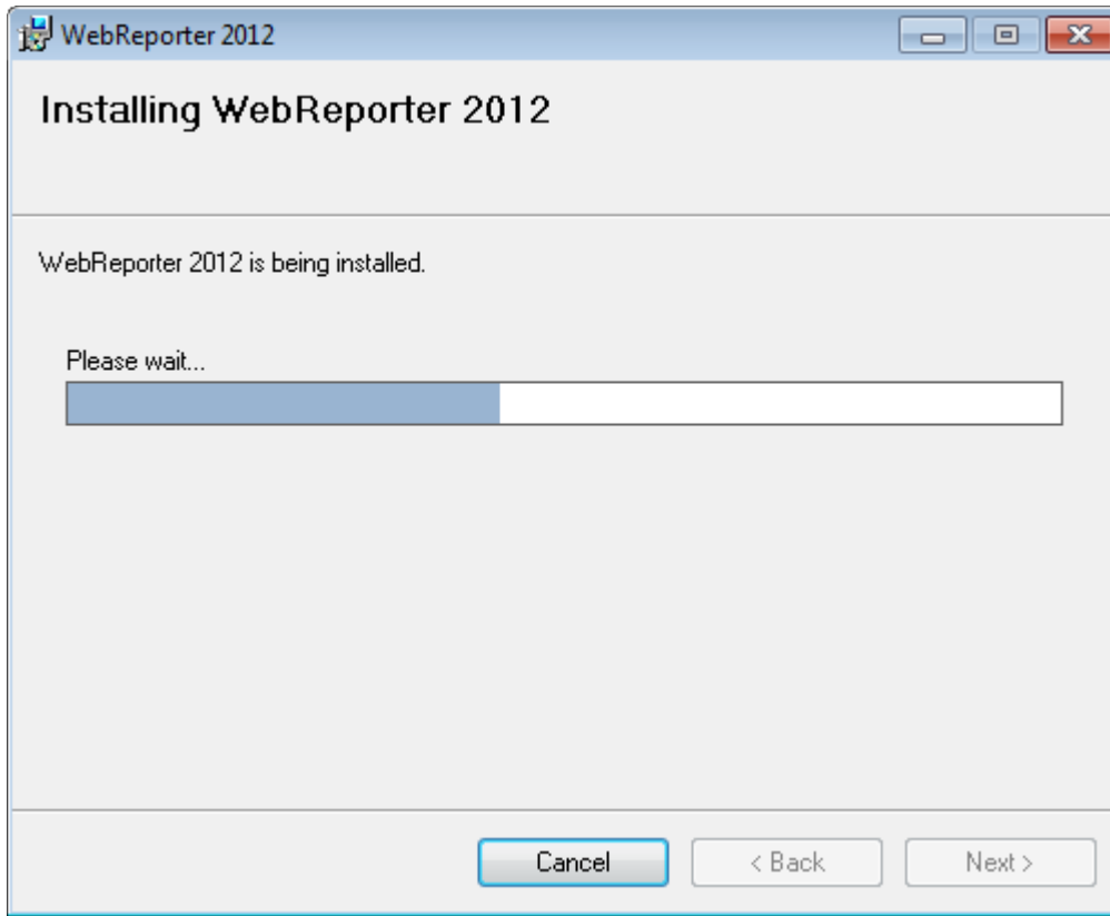
图 8 - 安装进程
