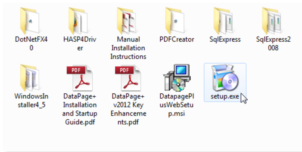
图 2 - Setup.exe 文件
